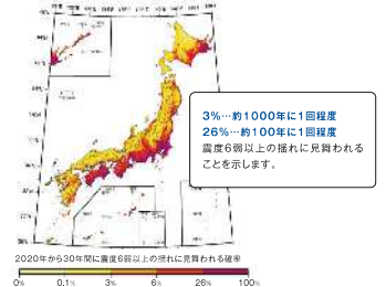
全国地震動予測地図2020年版 (地震調査研究推進本部)
